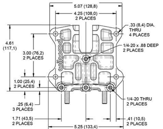
VIEW A-A
